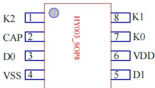
Sop8
