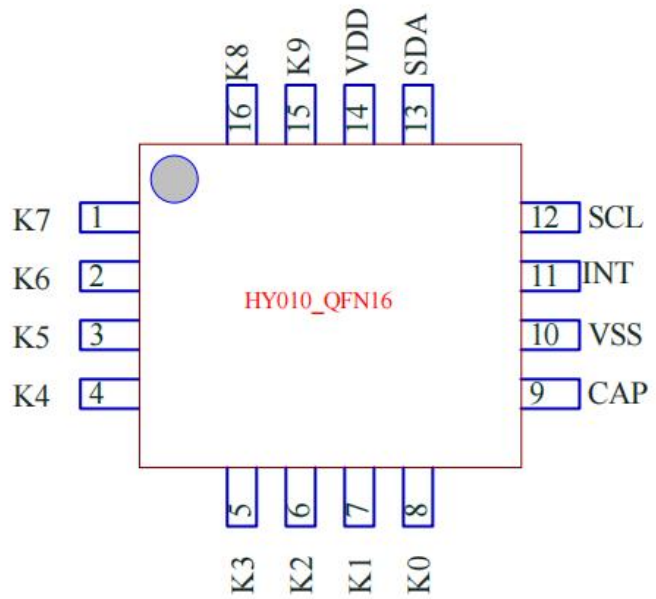
QFN16
