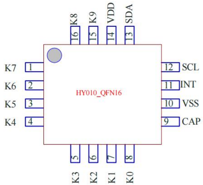
QFN16
